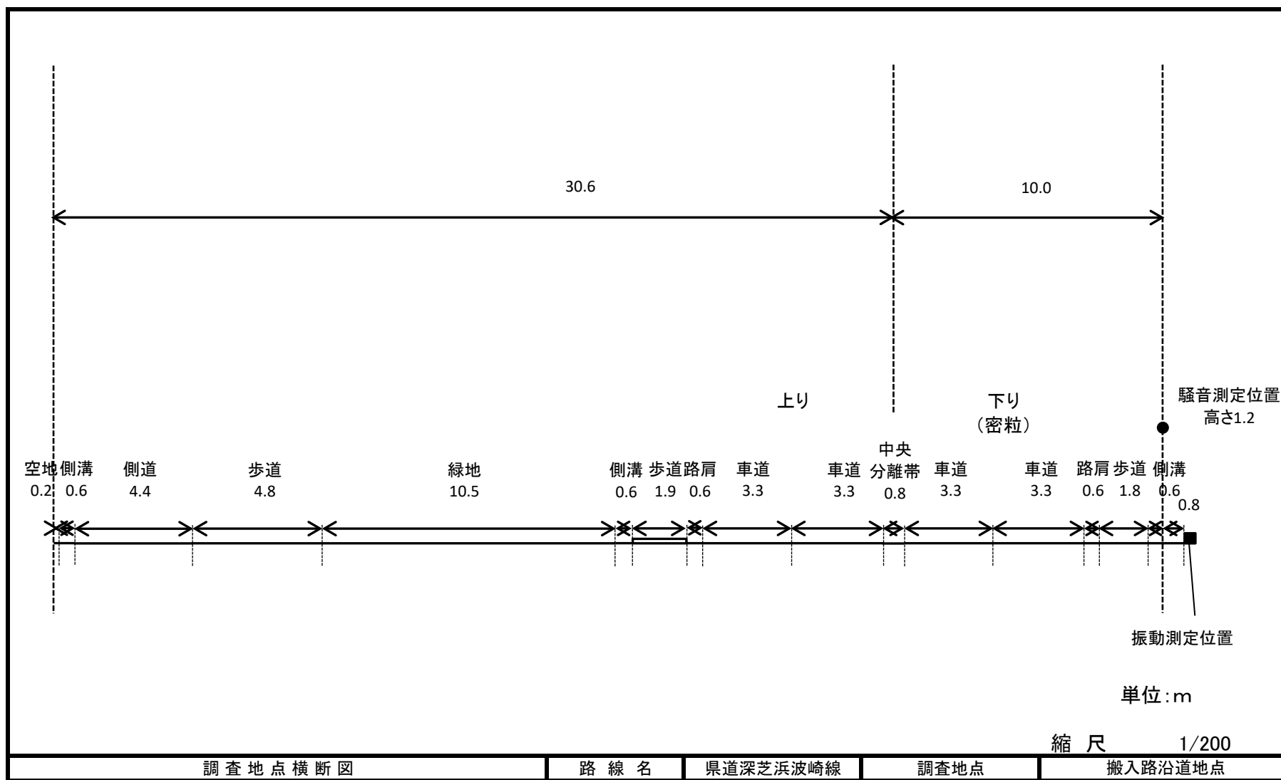
調査地点横断面図
